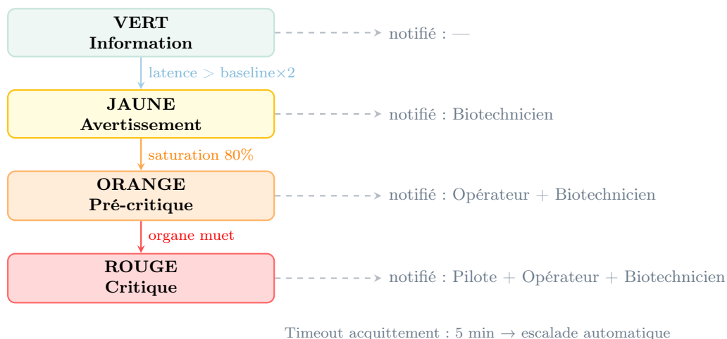
FIGURE 5 – Protocolum Vigilis : escalade des alertes et rôles notifiés. Si une alerte n’est pas acquiescée dans le délai, elle est automatiquement escaladée au niveau supérieur.
