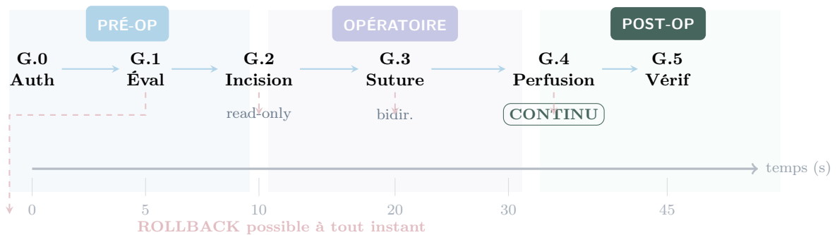
FIGURE 2 – Chronologie d'une greffe numérique. Trois phases distinctes : PRÉ-OP (préparation, 0-5s), OPÉATOIRE (transplantation read-only, 5-10s), POST-OP (perfusion continue et vérification). Le rollback est possible à tout instant.
