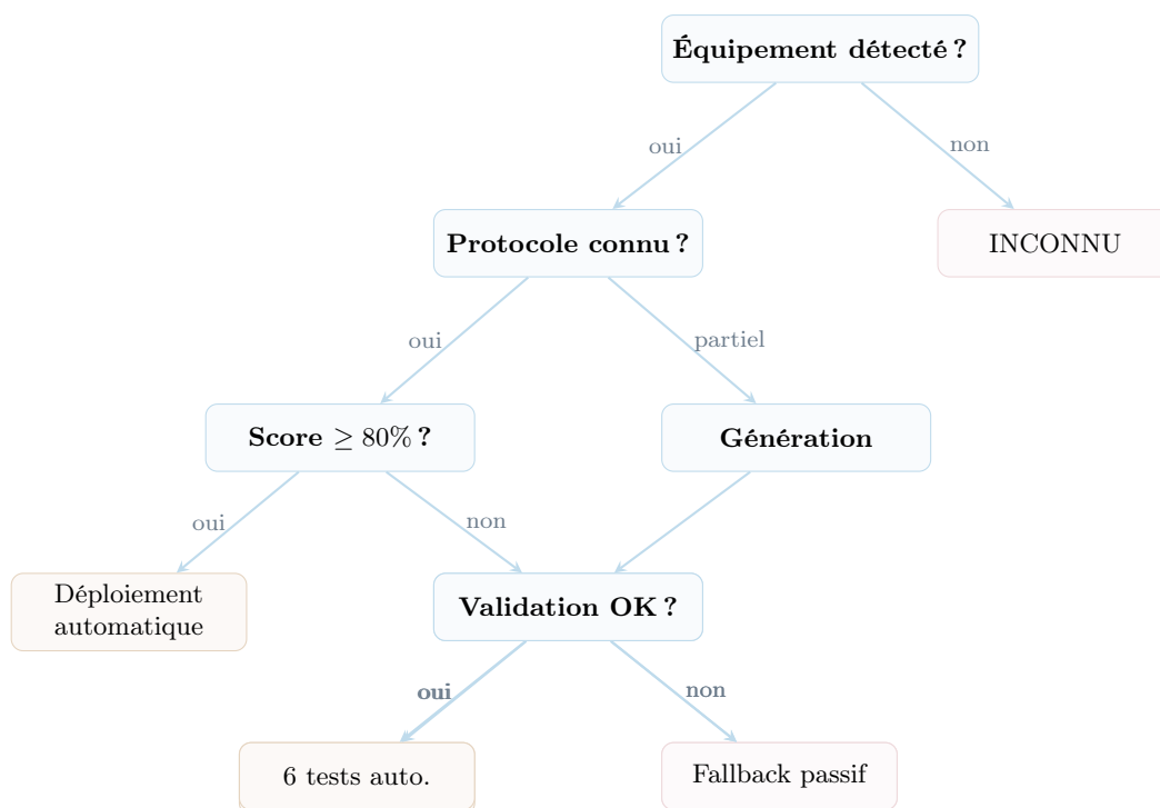
FIGURE 8 – Arbre de décision des connecteurs auto-adaptatifs. Le pipeline aboutit soit à un déploiement automatique ( \geq 80\% ), soit à une proposition humaine ( 50\text{--}80\% ), soit à un mode passif par proxy ( < 50\% ).
